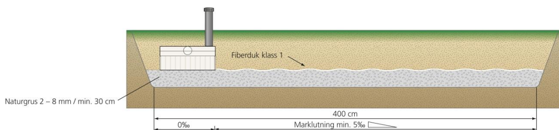
Typritning 4
