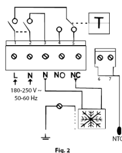
Koblingsskjema for kjøling
