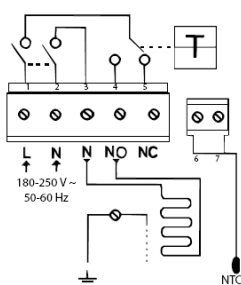
Koblingsskjema for varme
