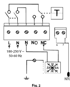
Koblingsskjema for kjøling
